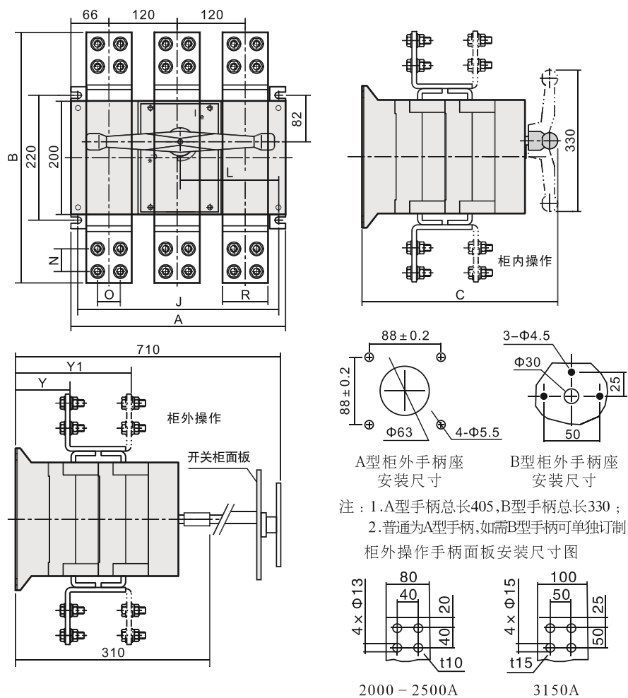
■ HGL-2000~3150A 隔离开关外形及安装尺寸
