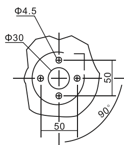
柜外手柄座安装尺寸
