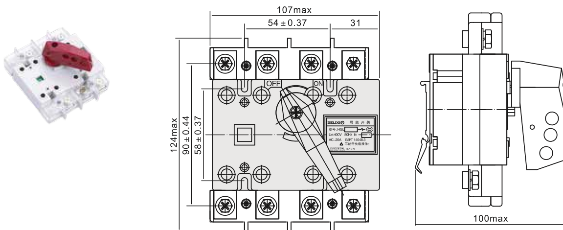
HGL、HGLi-80~100/3(4) 隔离开关外形及安装尺寸
