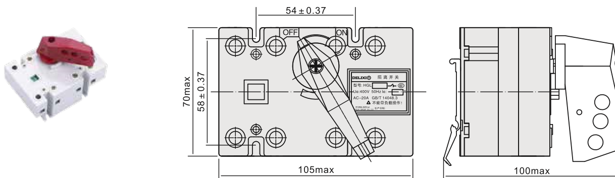
HGL、HGLi-16~63/3(4) 隔离开关外形及安装尺寸
