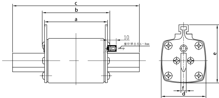
RT16A刀型触头熔断体的外形尺寸图
