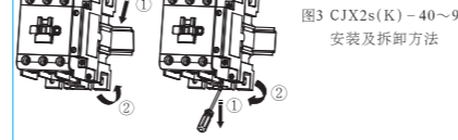
图3 CJX2s(K)-40~95 安装及拆卸方法
