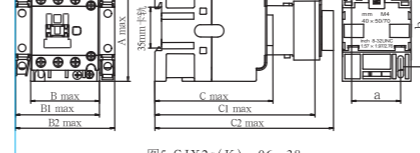
图5 CJX2s(K)-06~38
