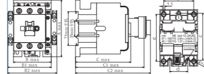
图6 CJX2s(K)-40~95
