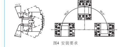
图4 安装要求
