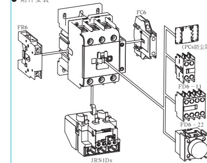
图9 附件安装示意图
