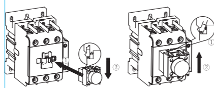
图12 空气延时头的安装 图13 空气延时头的拆卸
