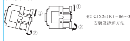
图2 CJX2s(K)-06~38 安装及拆卸方法
