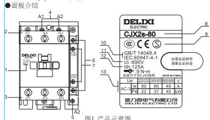
图1 产品示意图
