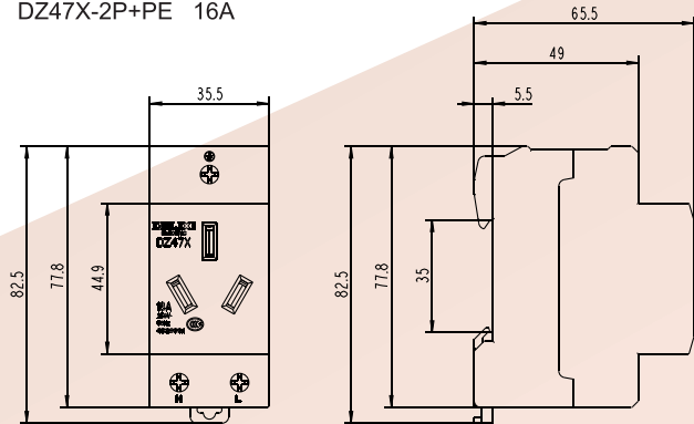
DZ47X-2P+PE 16A
