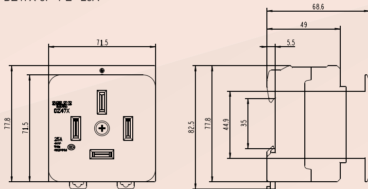
DZ47X-3P+PE 25A
