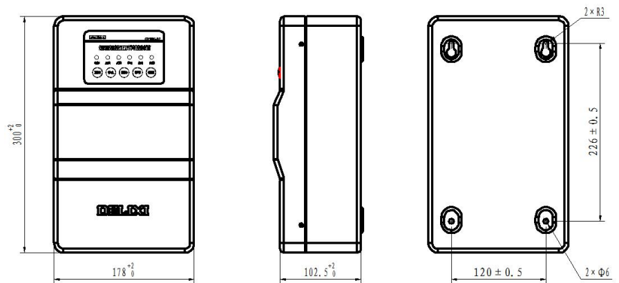
CDZFK 远程遥控正反转控制箱外形及安装尺寸
