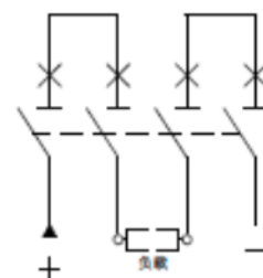
图 3 (4P 外形)
