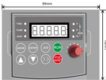
操作键盘安装尺寸
