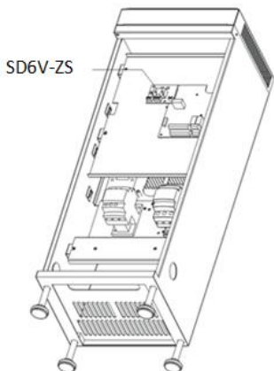
SD6V-ZS 安装方式
