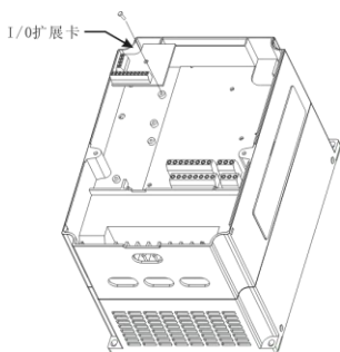
I0 扩展卡安装方式
