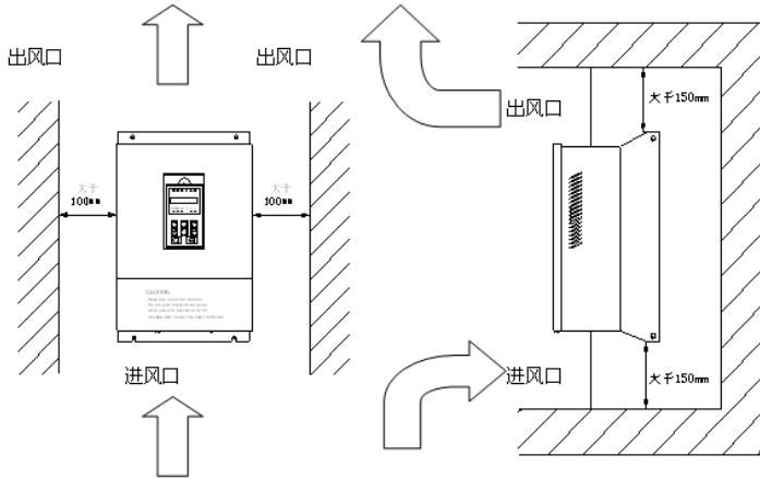
SD6 系列变频器的安装空间
