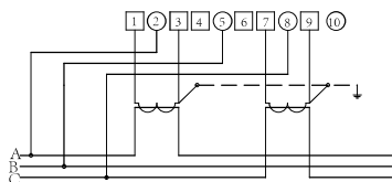
■ 三相三线电流互感器接入式接线图
