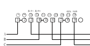
■ 三相三线直接接入式接线图
