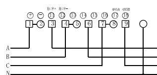
■ 三相四线直接接入式接线图
