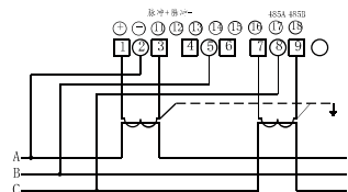
■ 三相三线电流互感器接入式接线图
