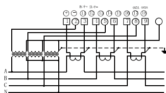
■ 三相四线电流、电压互感器接入式接线图
