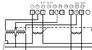
■ 三相三线电流、电压互感器接入式接线图
