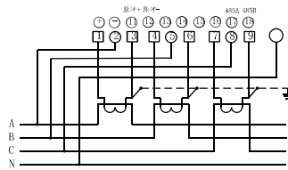
■ 三相四线电流、电流互感器接入式接线图
