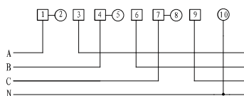
■ 三相四线直接接入式接线图
