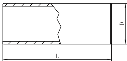
10×38、14×51、22×58直通铜管的外形尺寸图
