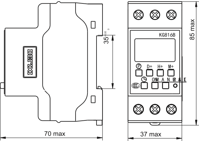
外形及安装尺寸(mm)
