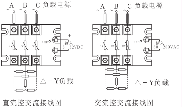
直流控交流接线图 交流控交流接线图
