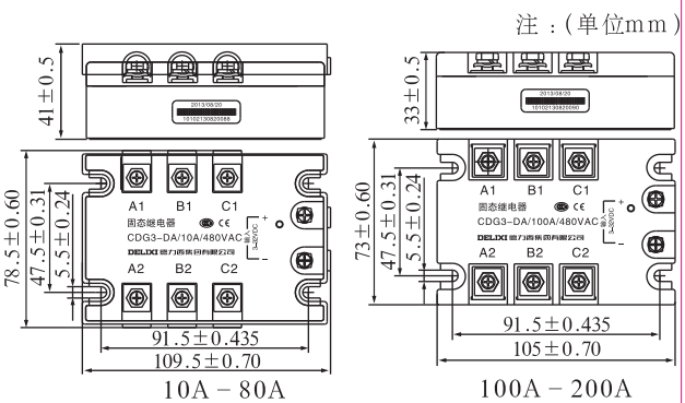
外形、安装尺寸
