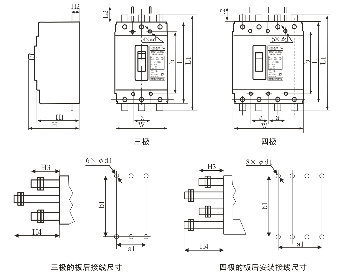
图1 断路器的外形尺寸和安装尺寸图
