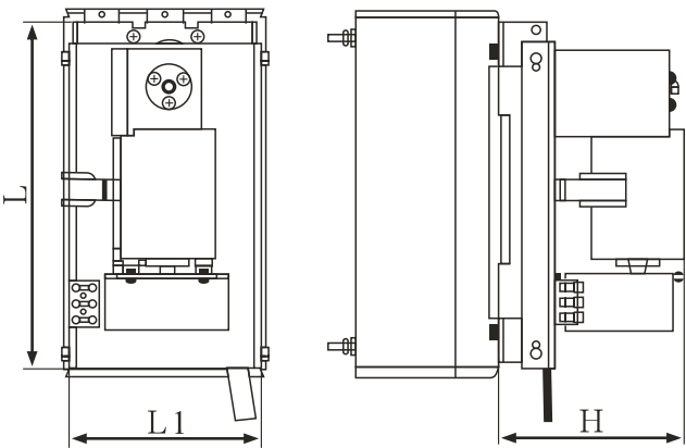
图2b DZ20-225、400、630、1250
