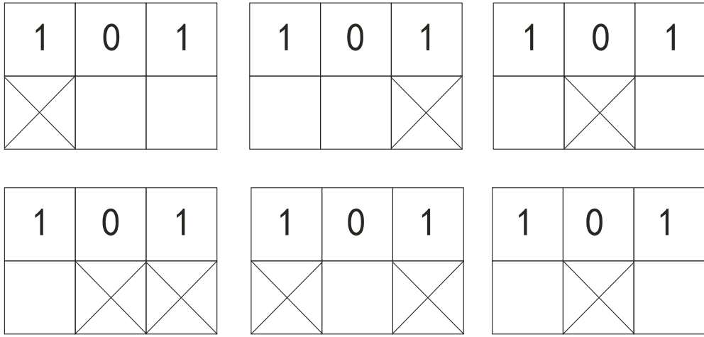
图2 LX10 - \frac{11}{12} 型行程开关每回路 可组成的关合表
