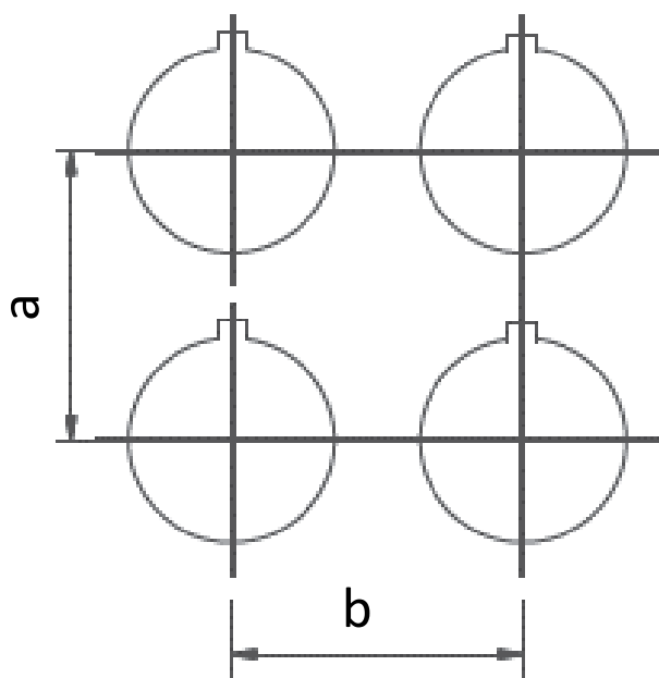
CDA9按钮开关安装中心距离尺寸表vs其他系列：mm 灰色填充表示该系列没有的型号
