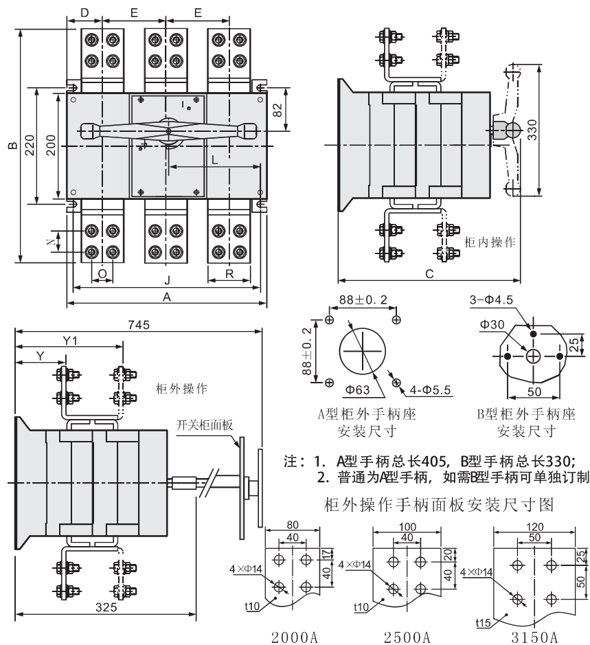
■ HGL-2000~3150A 隔离开关外形及安装尺寸
