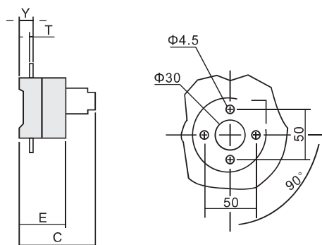
柜外手柄座安装尺寸
