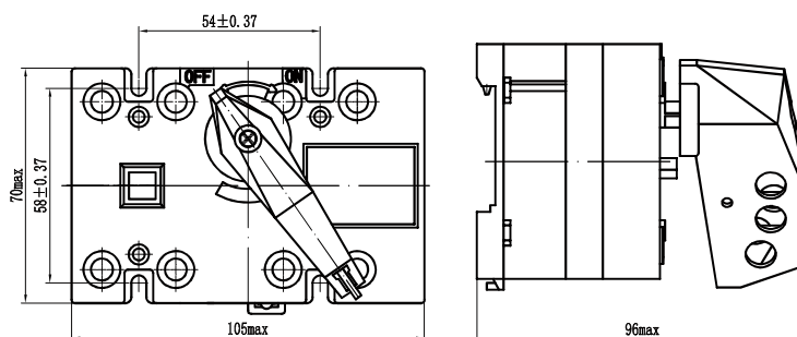
HGL、HGLi-16~63/3(4) 隔离开关外形及安装尺寸
