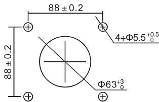
A 型柜外手柄座安装尺寸
