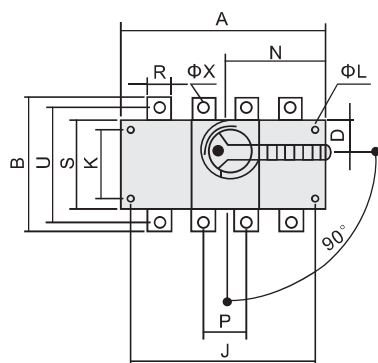
HGL、HGLi-125~630A 直接操作
