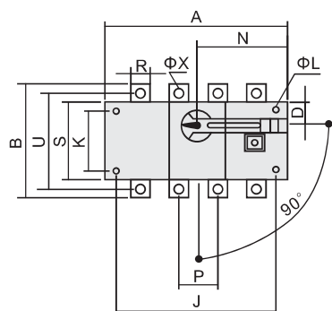
HGL、HGLi-125~630A 直接操作
