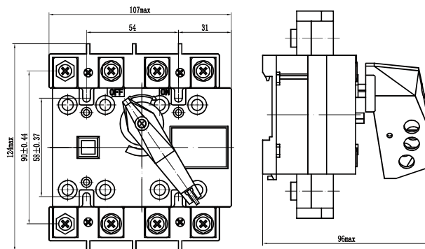
HGL、HGLi-80~100/3(4) 隔离开关外形及安装尺寸
