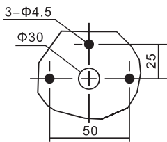
B 型柜外手柄座安装尺寸
