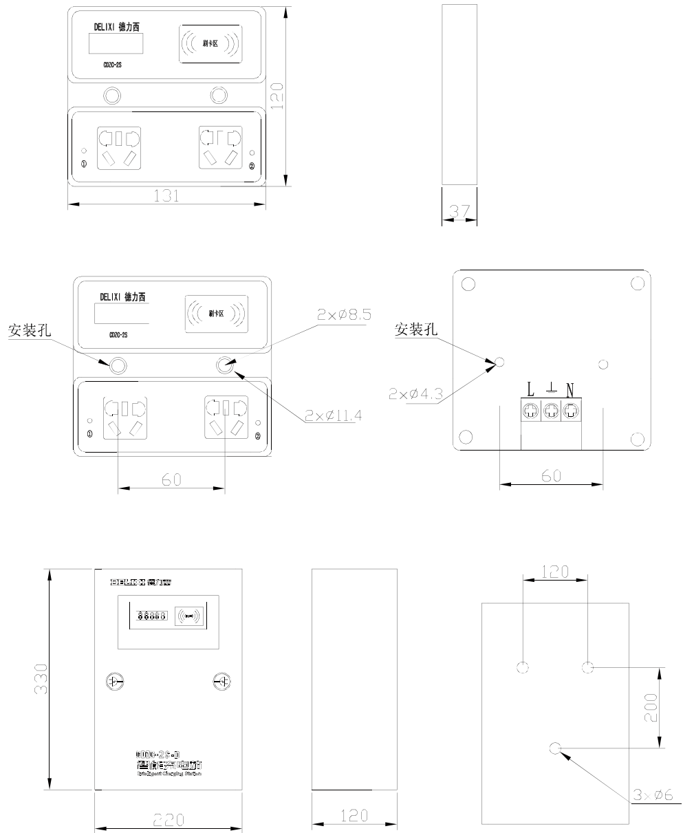
外形及安装尺寸 (mm)
