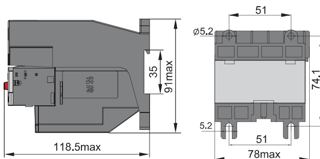
CDR9i-95 独立安装
