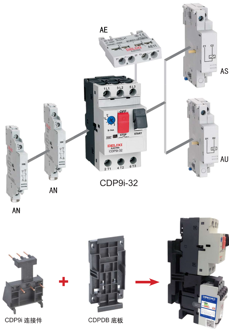
附件安装示意图
