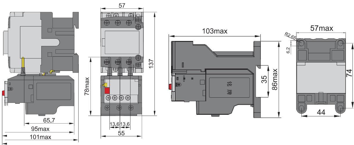
CDR9i-32 组合安装
