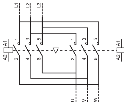
CDC9i-115N~630N (水平安装, 机械互锁)
