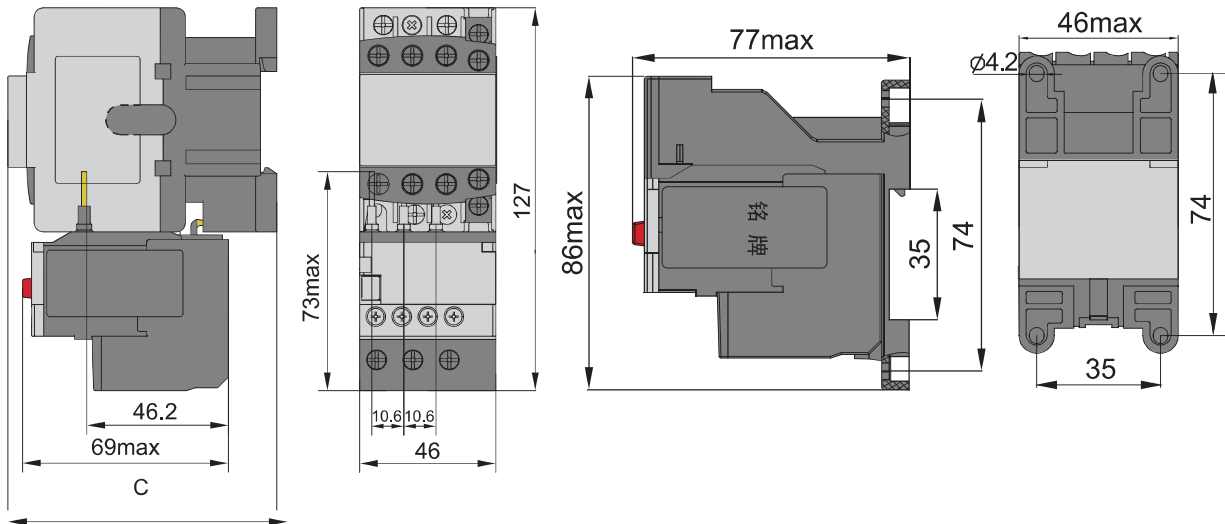
CDR9i-18 与 CDC9i-09、12、18 组合安装
