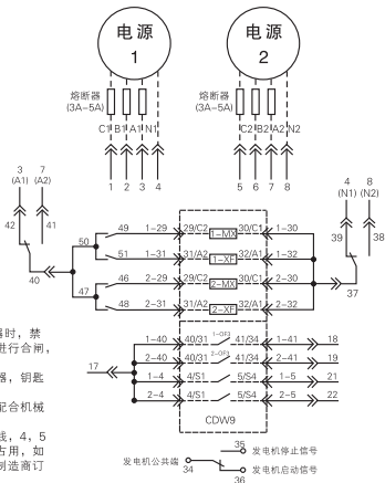
6.2 接线示意图
