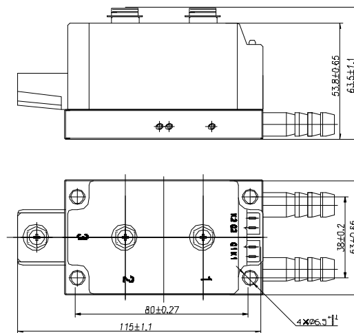
MTC-251A、301A/1600V/S 水冷系列晶闸管模块
