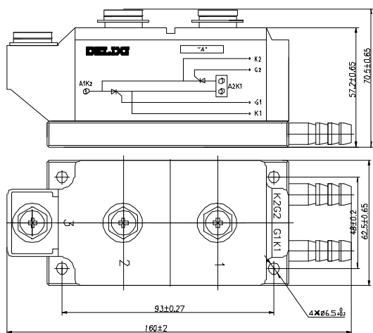
MTC-800A、1000A/1600V系列晶闸管模块
