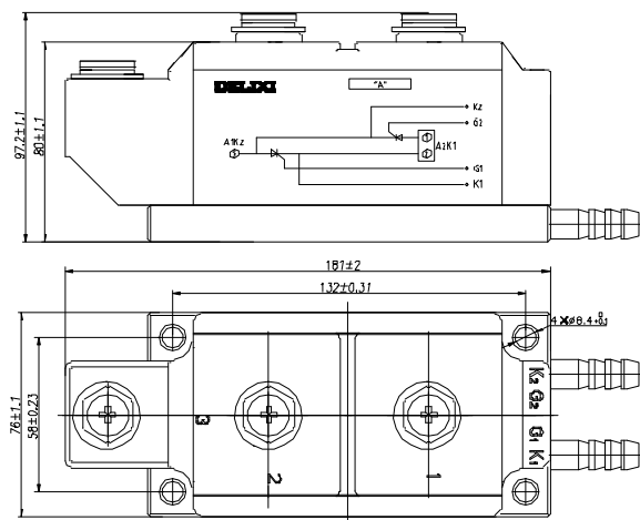
MTC-800A、1000A/1600V/S 水冷系列晶闸管模块
