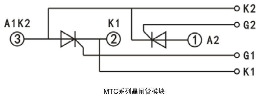
电路图
