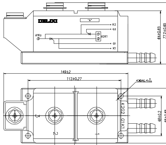
MTC-600A/1600V/S 水冷系列晶闸管模块
