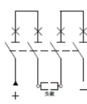
图 3 (4P 外形)
