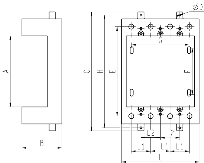
插入式板后孔位图
