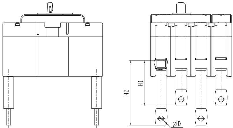
CDM6i 400~800 安装尺寸图
