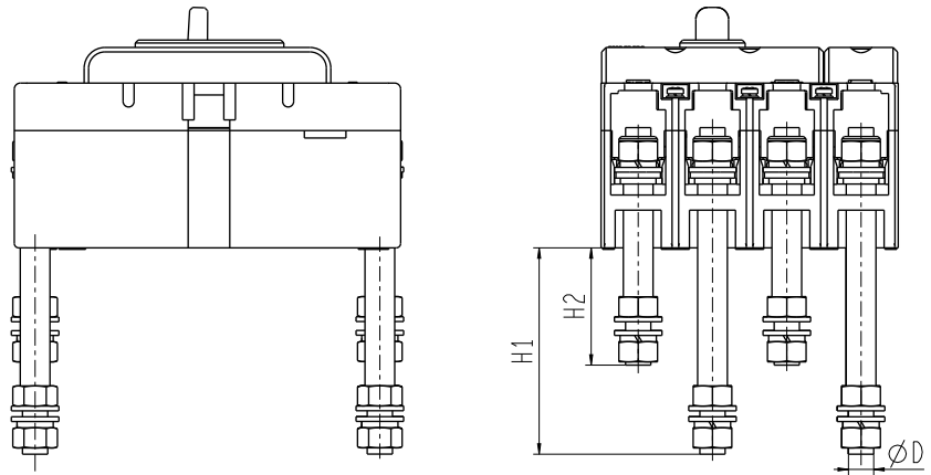
CDM6i-63~250 安装尺寸图
