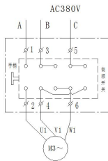
QS-30倒顺开关控制电机接线图
