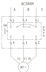
QS-15倒顺开关控制电机接线图
