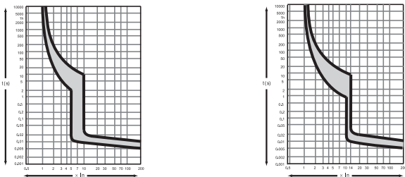
图1 C型热/电磁脱扣特性曲线
