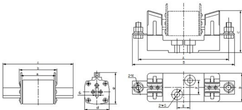
图 3 CDRS1 插入式熔断器的外形尺寸
