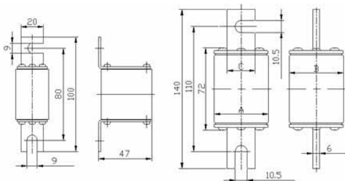
图 1 CDRS1-00 熔断器的外形及安装尺寸 图 2 CDRS1-1~3 熔断器的外形及安装尺寸
