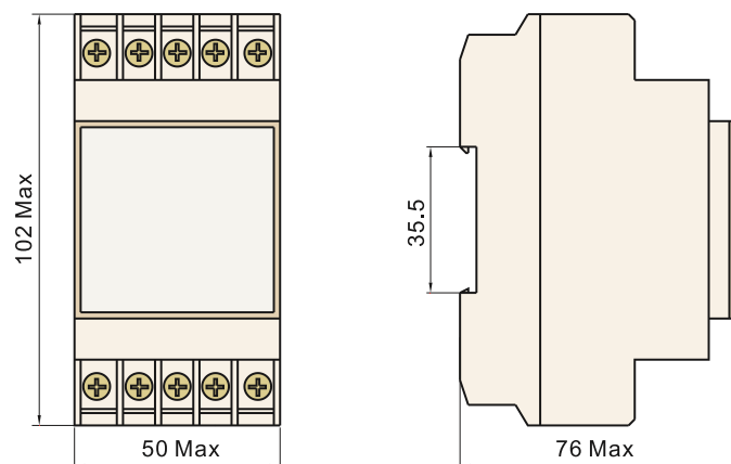
外形及安装尺寸(mm)
