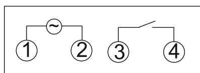
接线图
