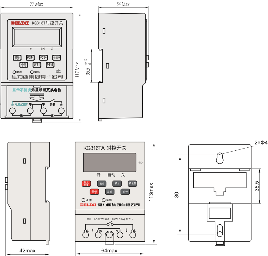
外形及安装尺寸(mm)
